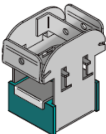
VibraFon CHP Super T60 ontworpen om vast te klikken aan vrijwel alle profielen op de markt, onaf- hankelijk van de profielhoogte, met beveiliging tegen ont- koppeling en foute montage
