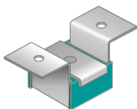
VibraFon CHP 1 Directe montage aan plafond d.m.v. 2 schroeven
