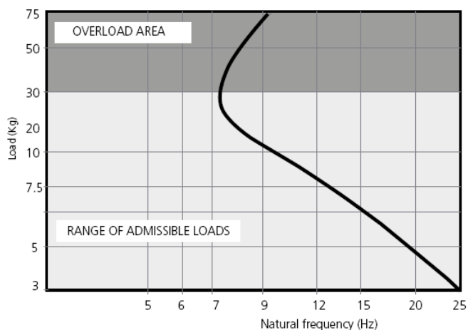
AFVEERFREQUENTIE Vibrafon CHP 30
