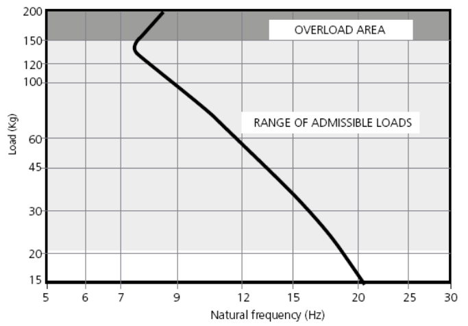
AFVEERFREQUENTIE Vibrafon CHP HD 150
