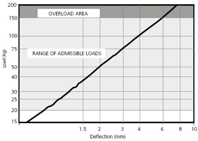
INVERINGSDIAGRAM Vibrafon CHP HD 150
