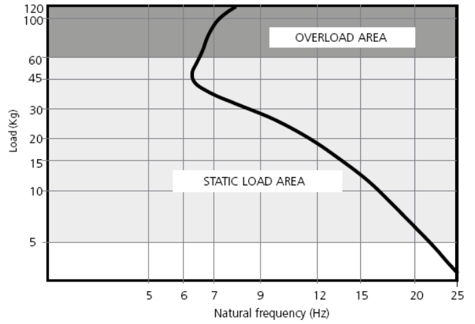
AFVEERFREQUENTIE Vibrafon CHPHD 60
