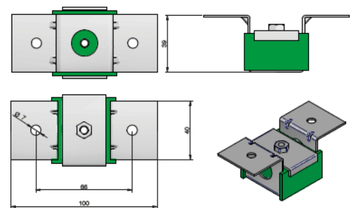
Hangende montage
