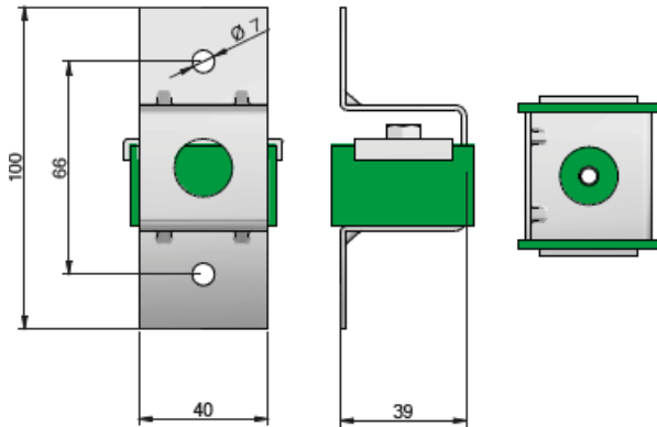
Zijdelingse montage
