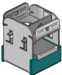
VibraFon CHP Super T47 ontworpen om vast te klikken aan vrijwel alle profielen op de markt, met in breedte verstelbare mounting
