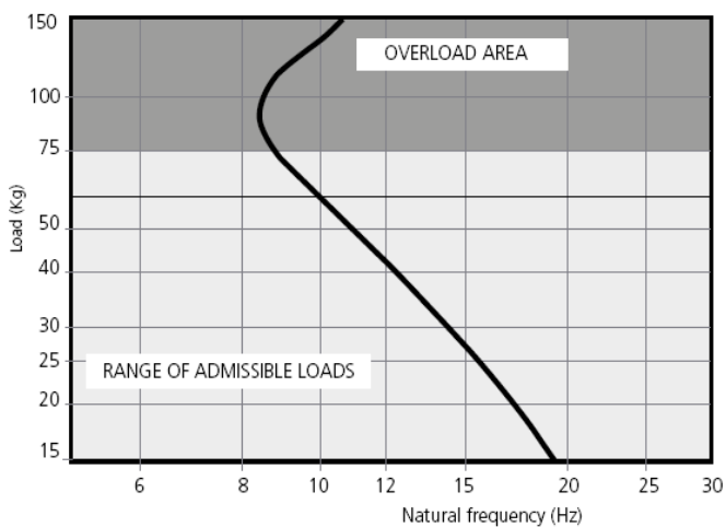
AFVEERFREQUENTIE Vibrafon CHP 75
