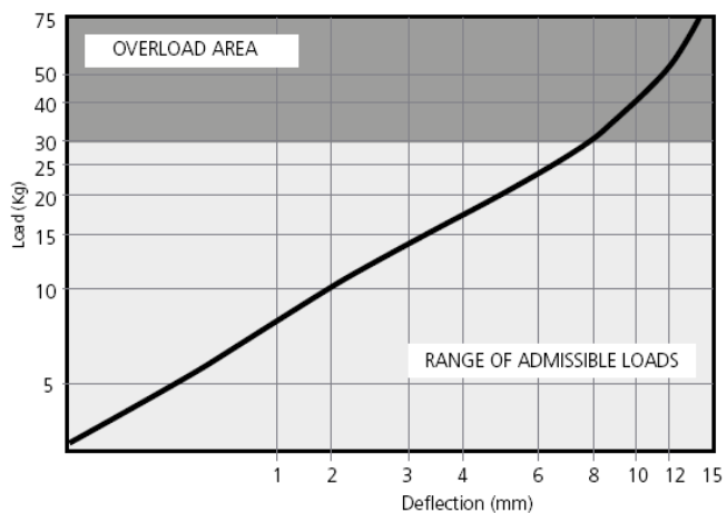
INVERINGSDIAGRAM Vibrafon CHP 30
